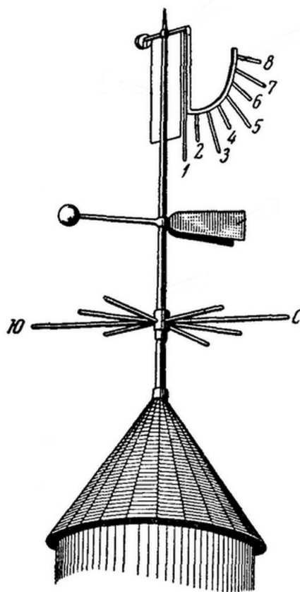
Рис. 9. Флюгер
